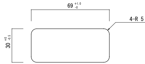
座板断面図 S=1/2
