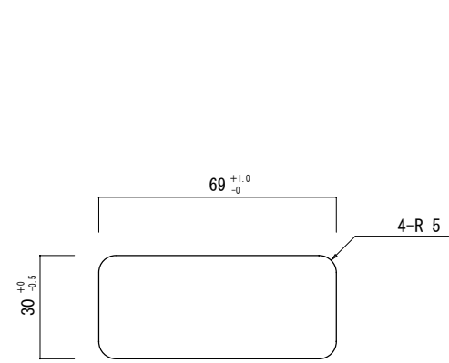
座板断面図 S=1/2
