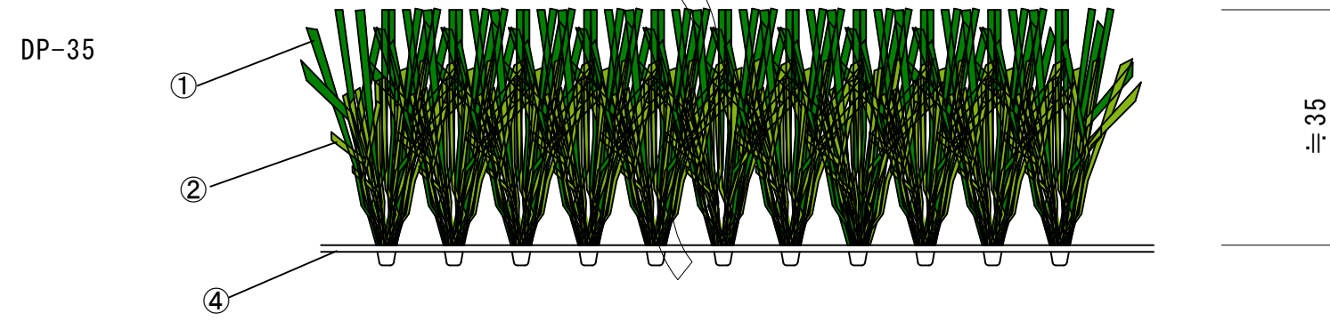
■ 横断面図a-a' (1/1)
