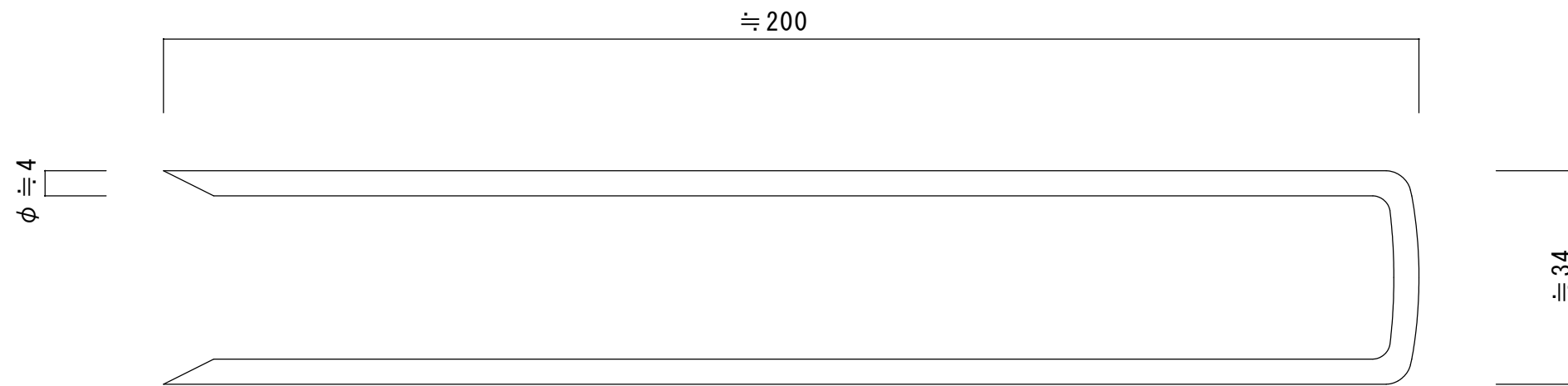
■コの字ピン（スチール製）
