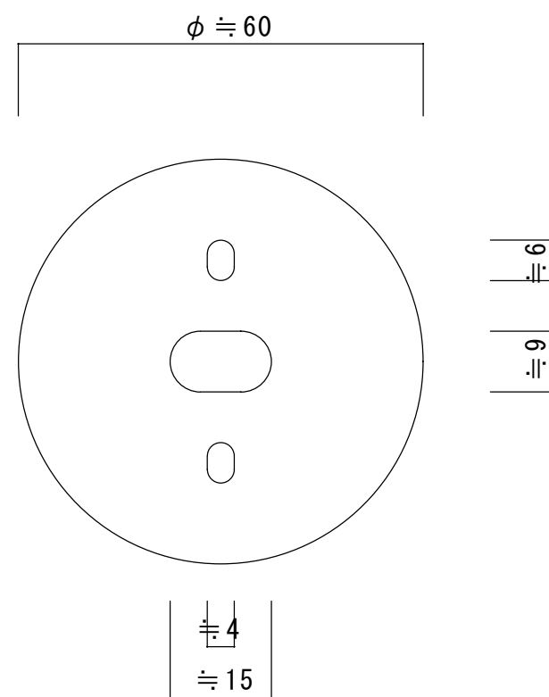
■防草シート用ワッシャー（ t \approx 2 ポリエチレン製）
