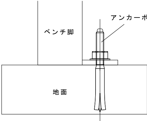
詳細A(アンカーボルト取付状態)
