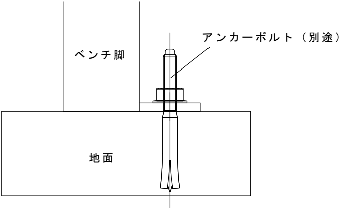
詳細A(アンカーボルト取付状態)
