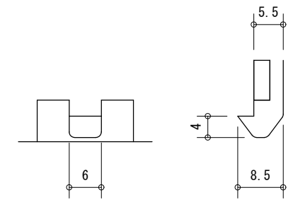
ジョイント (+)
