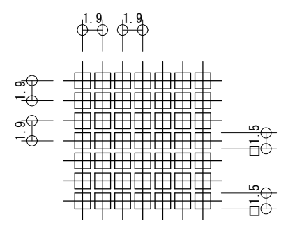
本体表面（シボ加工）詳細 S=2/1
