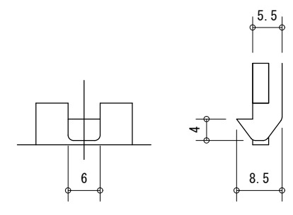
ジョイント (+)
