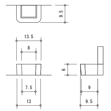
ジョイント (-)
