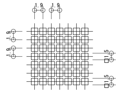
本体表面（シボ加工）詳細 S=2/1
