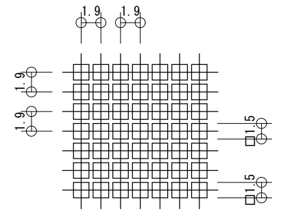
本体表面（シボ加工）詳細 S=2/1
