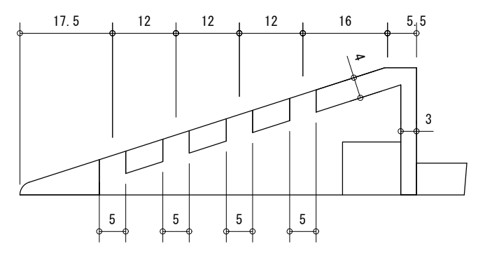
SECT A-A'
