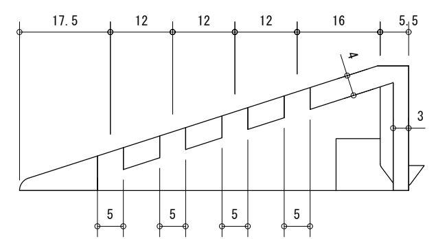
SECT A-A'
