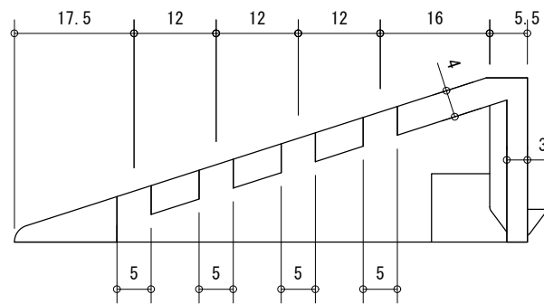
SECT A-A'
