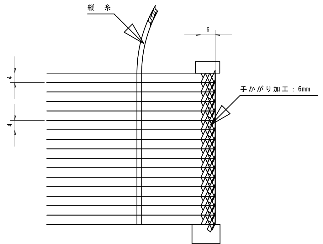
A部詳細（S=1／1）
