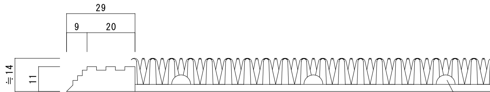
カール部断面図S=1/1
