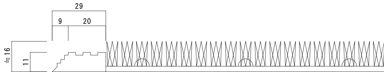
ストレート部断面図S=1/1
