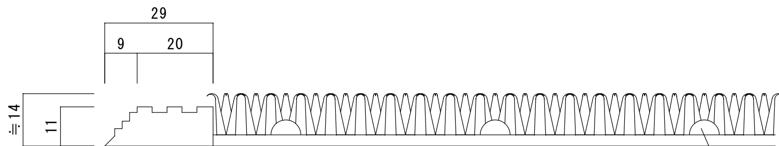
断面図S=1/1
