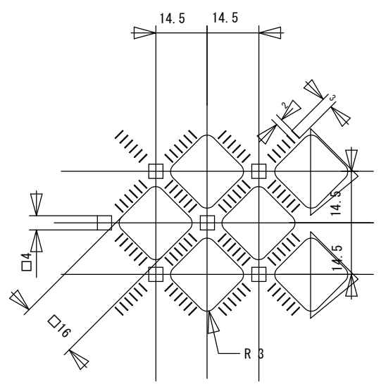
A部詳細 (S=2/3)
