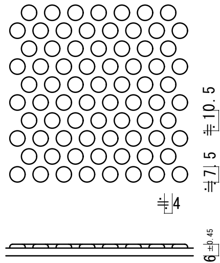
部分形状図 (1/2)
