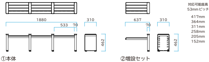
①本体 245-0100 (組立例) 組立例：座高/417mm・311mm・205mm
